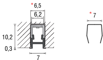
6010001 Clip di fissaggio (incluso) Fixing clip (included) Befestigungsclip (inbegriffen)
